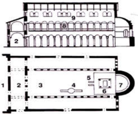
Resim 23: Konstantinopolis ve çevresindeki Erken Hıristiyanlık dönemine ait bir bazilikanın plan ve kesiti: 1. Avlu; 2. Narteks (Ön mekan); 3. Naos (cemaat mekanı); 4. Ambonun yeri; 5. Templon (altar odasını sınırlayan); 6. Kiborionlu altın yeri; 7. Synthrononlu apsis; 8. Galeri; 9. Işık kati. (Koch 2007. s.39 Res.14)
