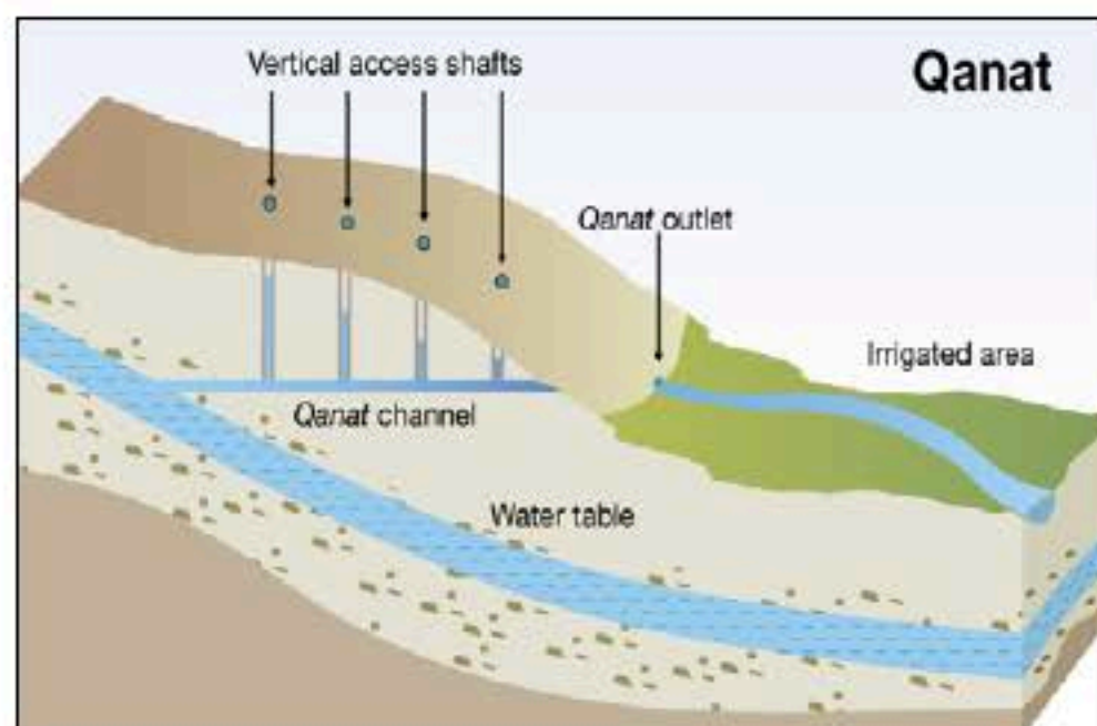
Fig. 3: the qanat system (SOURCE PRAVETTONI, 2010). Fig. 3: il sistema di qanat (da PRAVETTONI, 2010).
